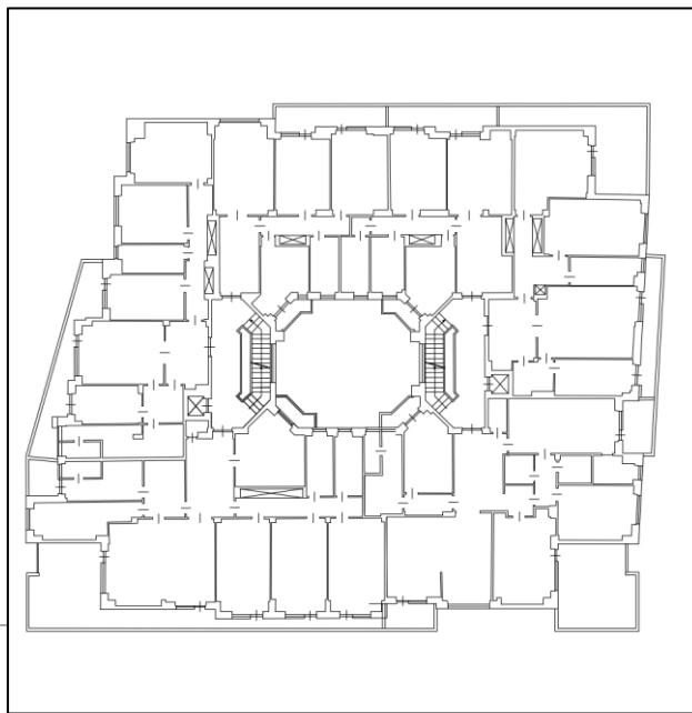
Pianta Piano Tipo- Stato dei luoghi
