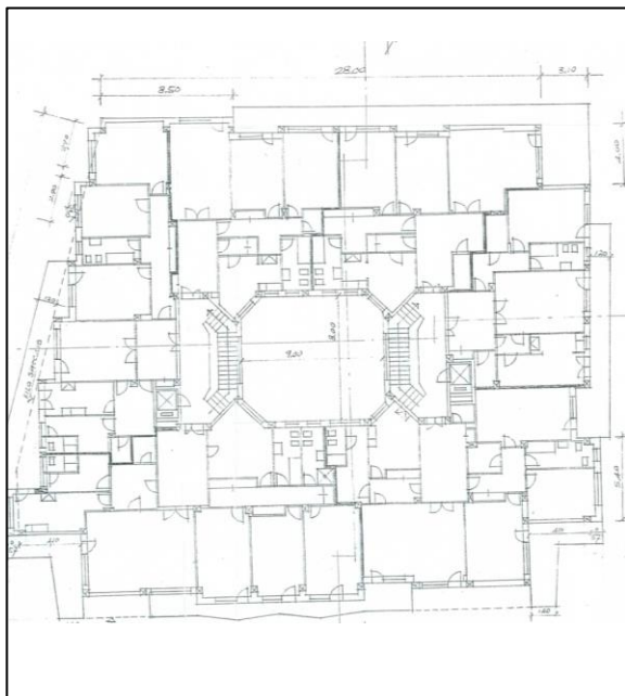
Pianta Piano Tipo- Licenza Edilizia
