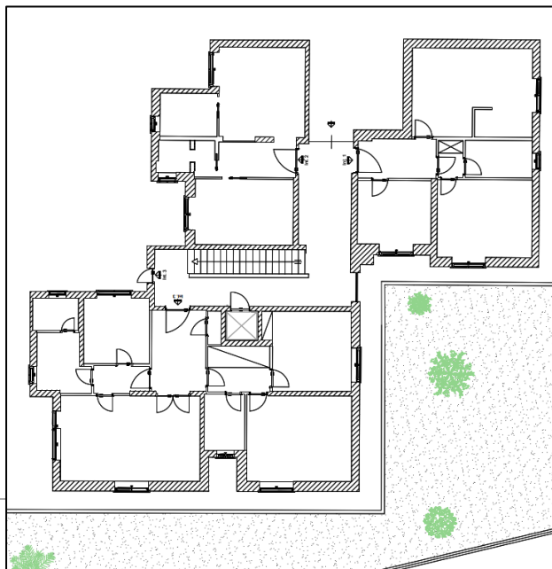
Pianta Piano Terra- Stato dei luoghi
