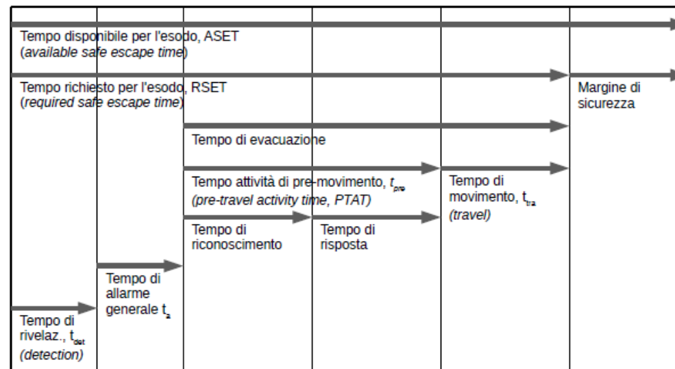
Illustrazione M.3-1: Confronto tra ASET ed RSET
