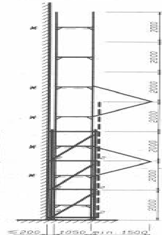
SEZIONE A-A
